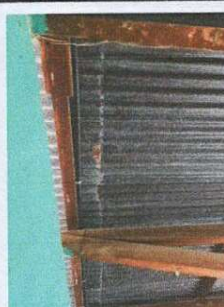
Foto 2: Sustitucion de estructura y cubierta de lamina por estructura metalica galvanizada, cargadores de 4"x4" y costanera de 4"x2" en aula 4
